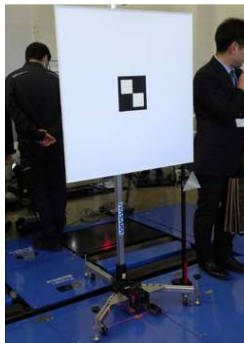
ターゲットボード用のスタンドとレーザー墨出し器・距離計等がセットになったエイミング用ターゲットスタンドセット。
